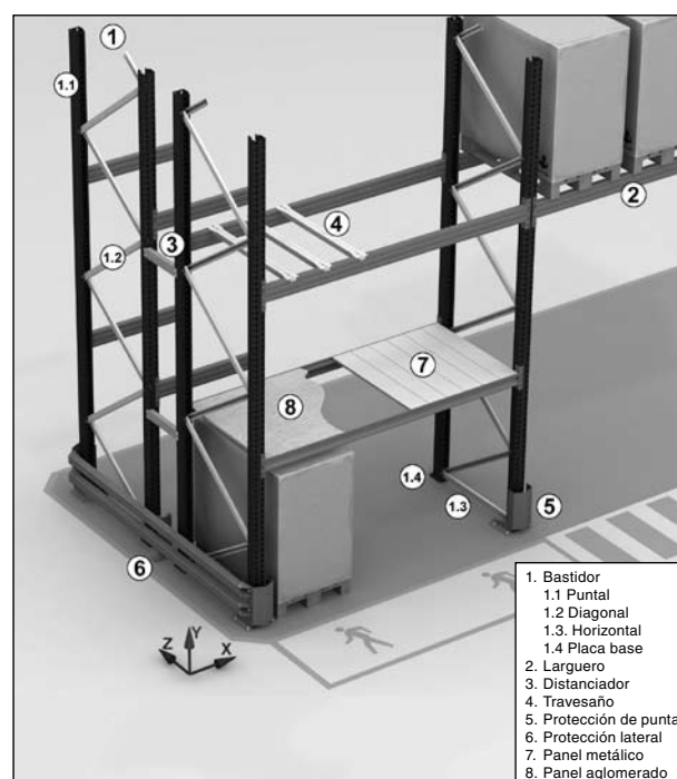
Figura 1. Componentes de la estantería
